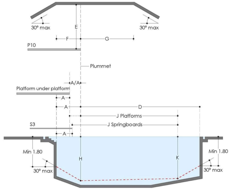
LONGITUDINAL SECTION
